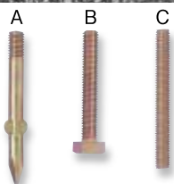
先とがり 六角ボルト 寸切
