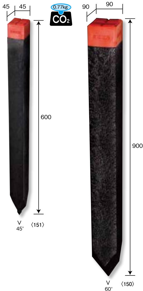
道路敷界杭45角
